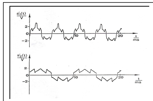
Sinyal demodulasi terdistorsi
