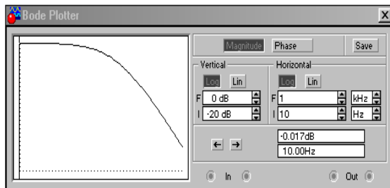
Gambar 2.16 Respon keluaran rangkaian Low Pass Filter aktif
