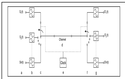
Gambar 2.1. Prinsip TDM dalam kasus PAM
