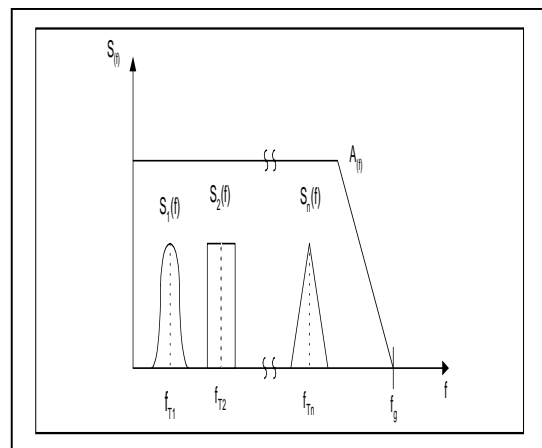
Gambar 2.2 : Konfigurasi kanal pada FDM
