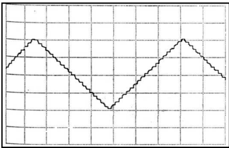
Sinyal Terkuantisasi (8 bit)
